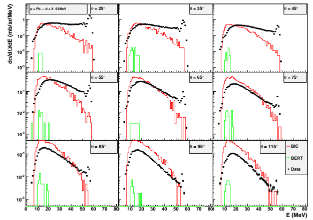
Fig. 9 p+Pb @ 63 MeV, deuteron production
