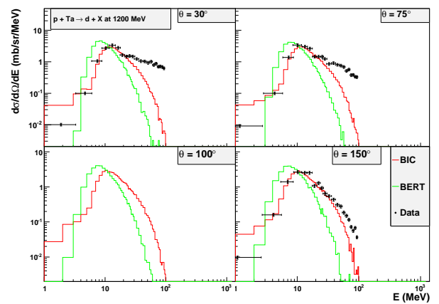
Fig. 10 p+Ta @ 1.2 GeV, deuteron production
